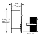
126- ADA Turn Piece
